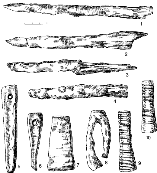
7 pav. Radiniai: 1–4 – peiliai iš k. Nr. 29, k. Nr. 73, k. Nr. 115, k. Nr. 107; 5–7 – galąstuvai iš k. Nr. 36, k. Nr. 73, k. Nr. 2; 8 – skiltuvas iš k. Nr. 52; 9–10 – adatinės atsiktinės ir iš k. Nr. 133
